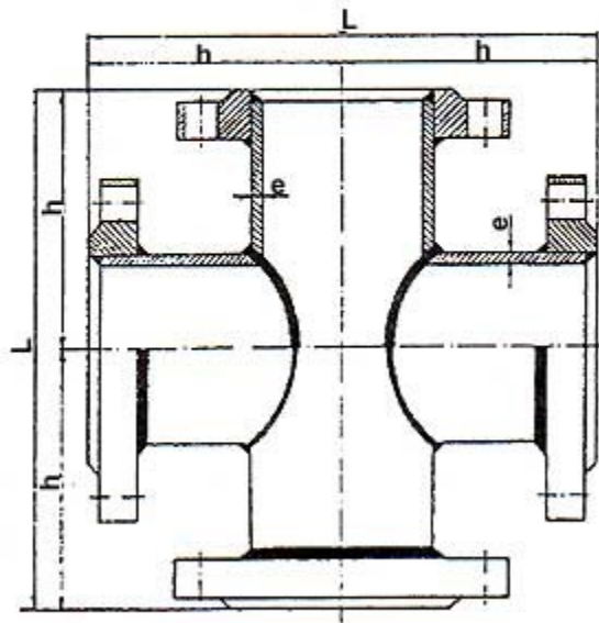
Krstasta račva sa prirubicama
