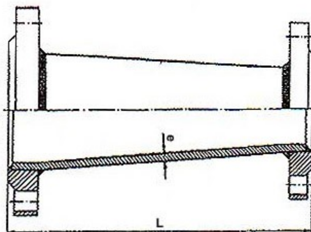
Redukcioni spojni element sa prirubicama
