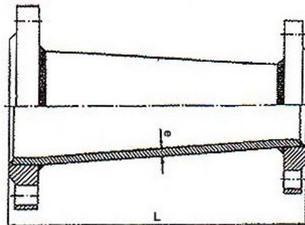
Redukcioni spojni element sa prirubicama
