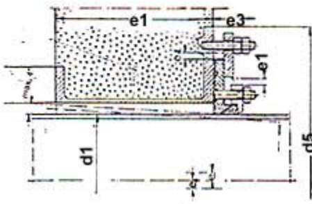
zidni provodnik za cevi sa elastičnim zaptivačem, poprečno pomerljiv
