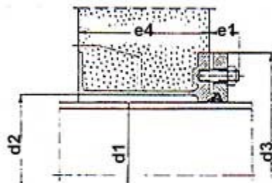
zidni provodnik za cevi sa elastičnim zaptivačem, navarenim vijcima kompaktne izvedbe
