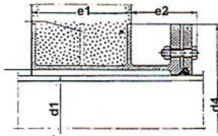
zidni provodnik za cevi sa elastičnim zaptivačem i prolaznim vijcima sa ispustom
